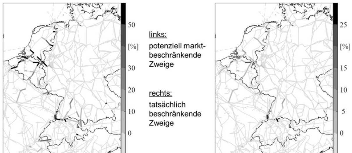
Analyse kritischer Netzelemente bei einer lastflussbasierten Marktkopplung
