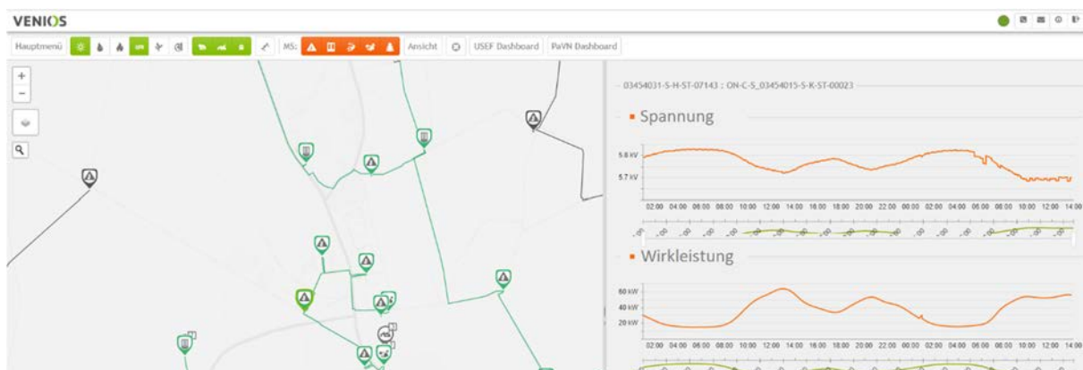
Visualisierung des Netzleitstandes mit VES zur prototypischen Demonstration im Feldtest
