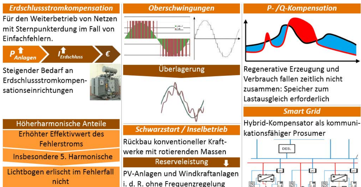
Systemdienstleistungen des Hybrid-Kompensators
