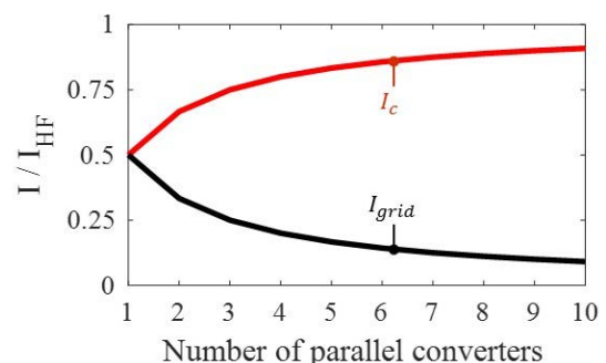
Aufteilung der Emission bei Schaltfrequenz zwischen dem Niederspannungsnetz und den Filterschaltungen der Geräte
