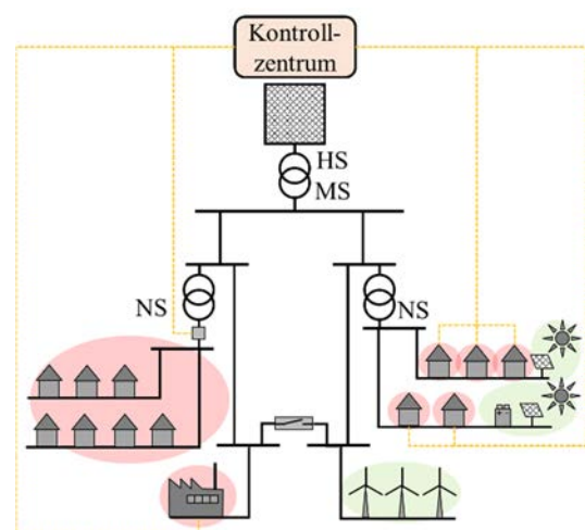
Selektives und dezentrales Lastabwurfkonzept
