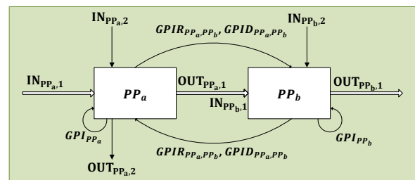
Darstellung der schematischen Produktionsprozesskette, welche für die simulativen Untersuchungen verwendet wurde.
