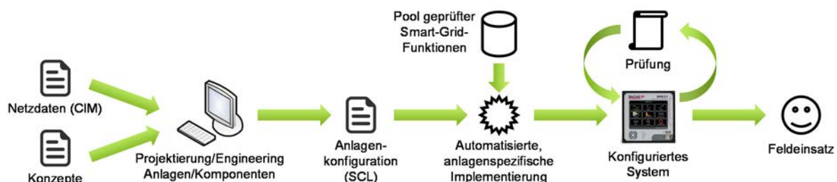
Gesamtkette aus Projektierung, Konfiguration und Prüfung des Systems
