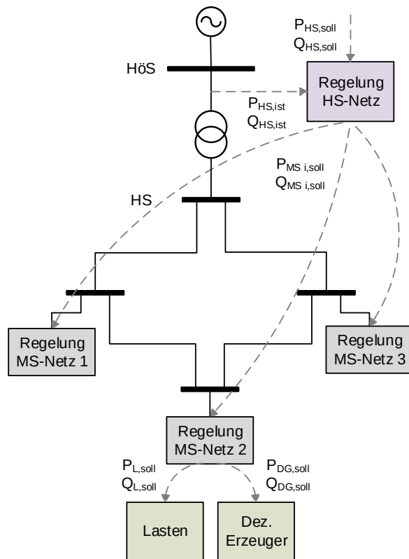
Verteilnetzregelung zur spannungsebenenübergreifenden Leistungskoordination
