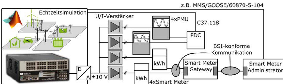
Die neue COMPASS Laborinfrastruktur: Smart Grid Simulation mit Smart Metern und PMU
