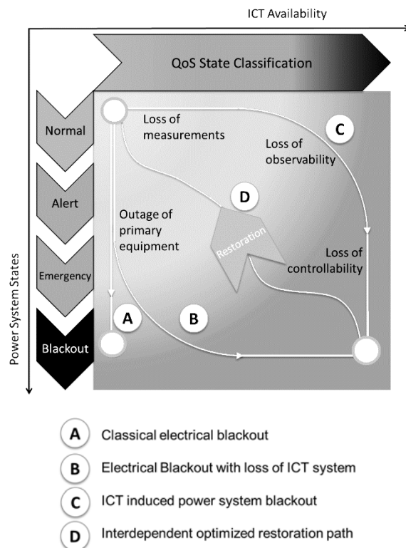
Kombiniertes Zustandsmodell für Energie und IKT
