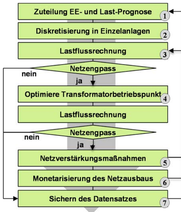
Gesamtkonzept zur automatisierten Bewertung des Netzausbaubedarfs im Verteilnetz
