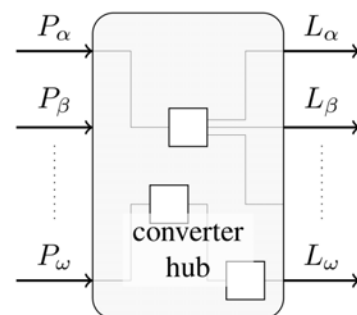
Eingangsleistungen und Ausgangsleistungen eines Energy Hubs
