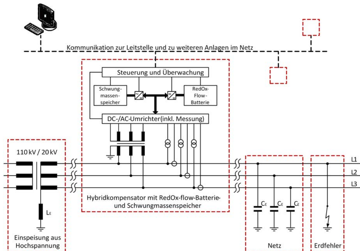
Blockschaltbild des multifunktionalen Hybridkompensators
