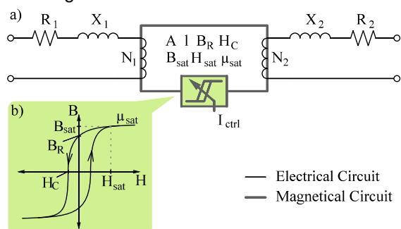
Modellierung der regelbaren Induktivität (a), Hysterese-Modell (b)
