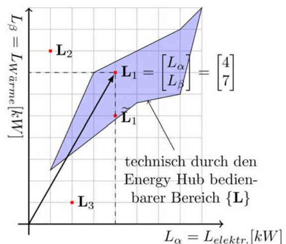
Qualitative Darstellung der Möglichkeit eines Energy Hubs, zwei Leistungsarten zu variieren
