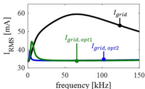
Stromaufnahme einer LED-Lampe mit (blau, grün) und ohne Optimierung (schwarz)
