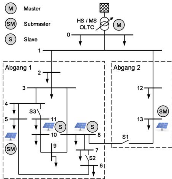
Mehrstufige Spannungsregelung
