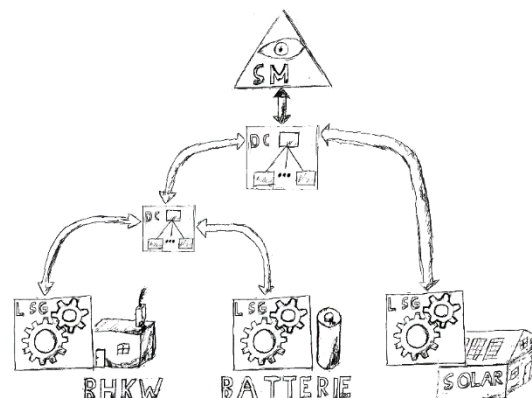
Struktur der dezentralen Einsatzplanung
