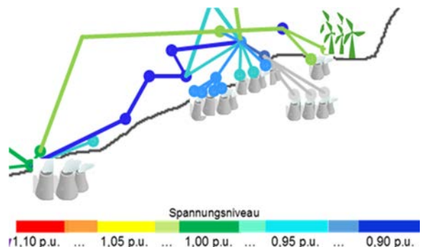
Übersicht des Spannungsprofils der kritischen Knoten im Süden
