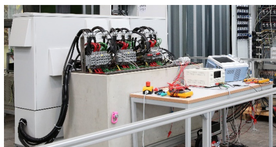
Längsreglerversuchsstand
