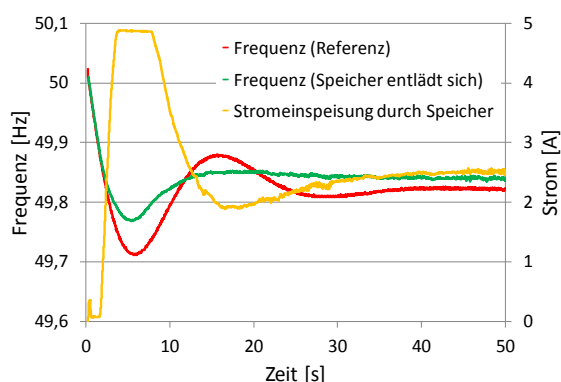
Schnelle Primärregelung durch Energiespeicher
