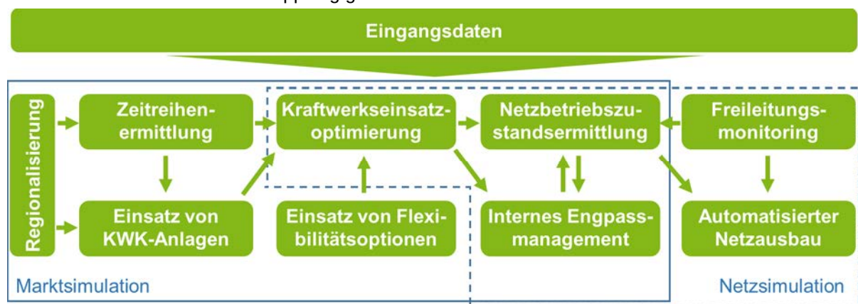
Markt- und Netzsimulationsumgebung MILES
