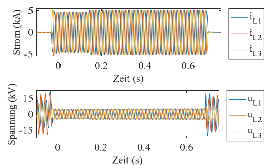
Störschrieb eines dreipoligen Kurzschlusses
