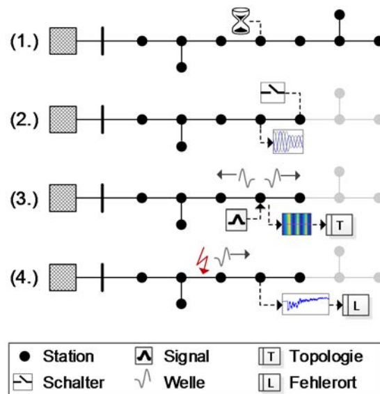
Konzept der autonomen, adaptiven Systemlösung zur Fehlerortung mit Wanderwellen
