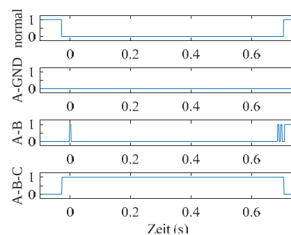
Klassifikationsergebnis mit SVM
